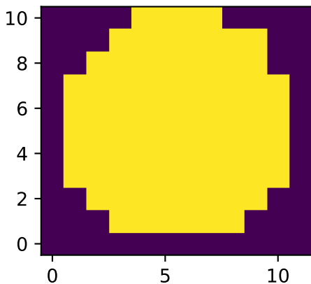
mode='center'
