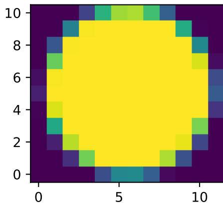
mode='exact'
